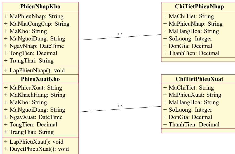
Hình 1: Sơ đồ lớp nghiệp vụ nhập xuất kho
